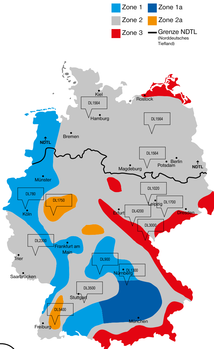
Abbildung: Beispiele örtlich erforderlicher DL-Klassen. Maßgebend sind Schneelastzone und Höhenlage. Auch die Dachform kann Einfluss haben. (hier Flachdach ohne Anhäufung)
